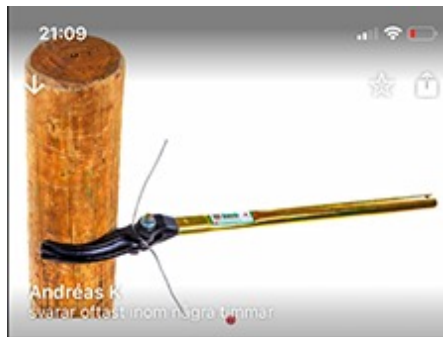
Stängselspännare/trådsträckare
